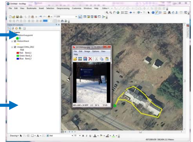
Desktop GIS
